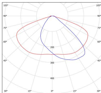
Исполнение «Ш8»
