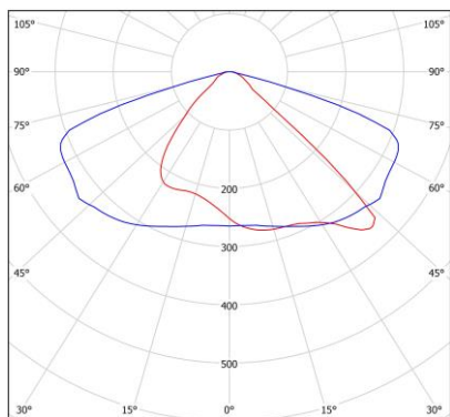
Исполнение «Ш7»
