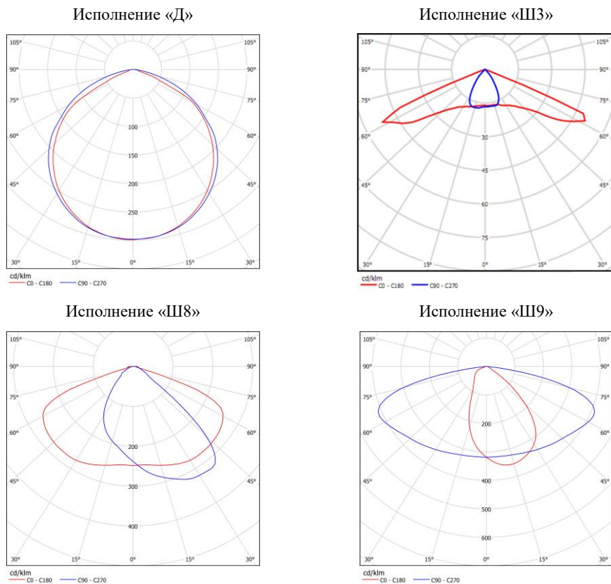
Рисунок 5 Типы КСС
