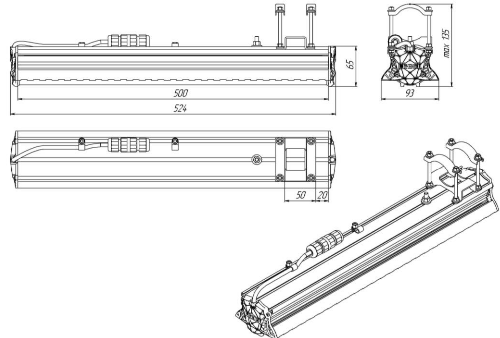
Рисунок 1 Габаритные размеры светильника «L-street 80 Turbine»
