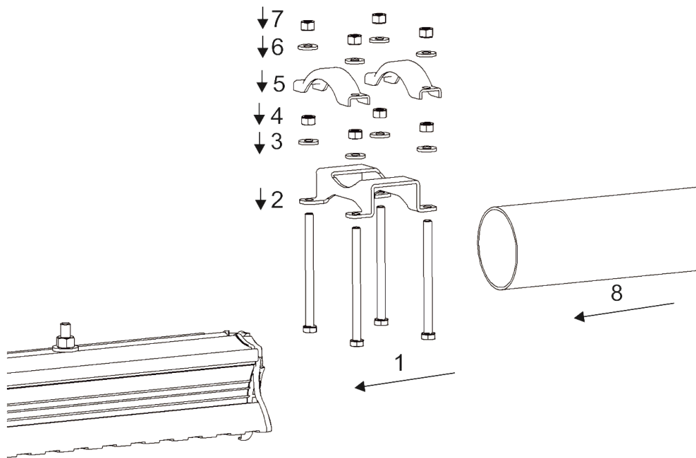
Рисунок 2 - Монтаж крепления
