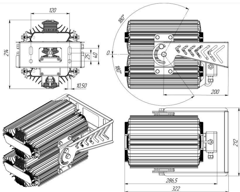
Рисунок 2 Светильник «L-lego 110» Поворотное крепление
